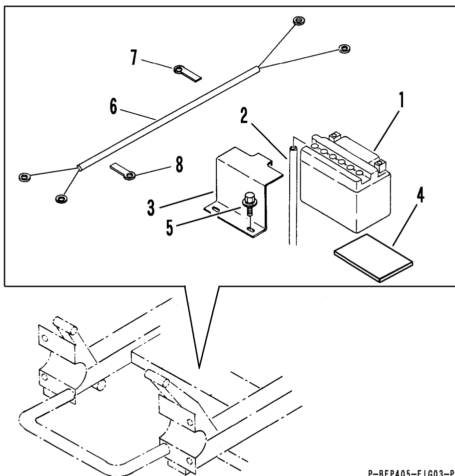
FIG 4 デンソウ (セルツキ) ELECTRIC EQUIPMENT (ELECTRIC STARTER)
