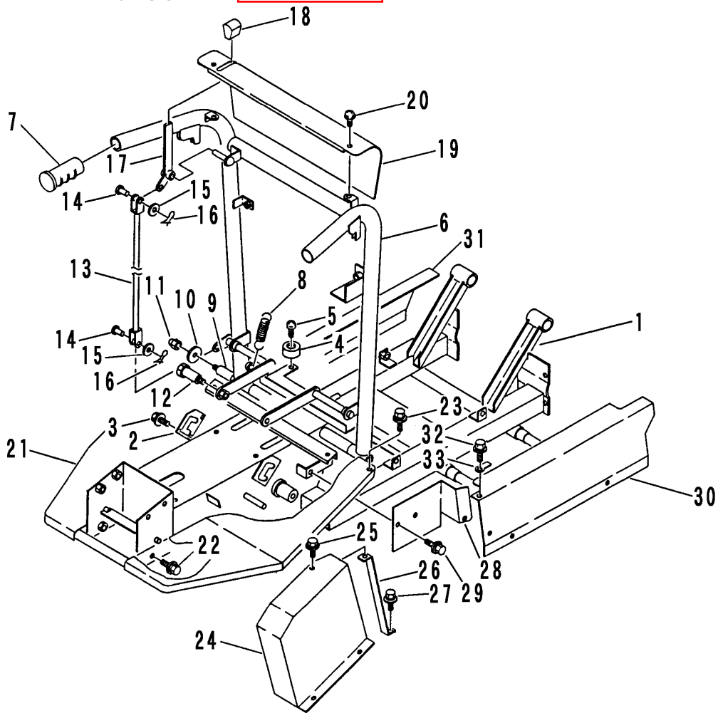
FIG 7 フレーム & カバー FRAME & COVER Serial Nr. -6112205
